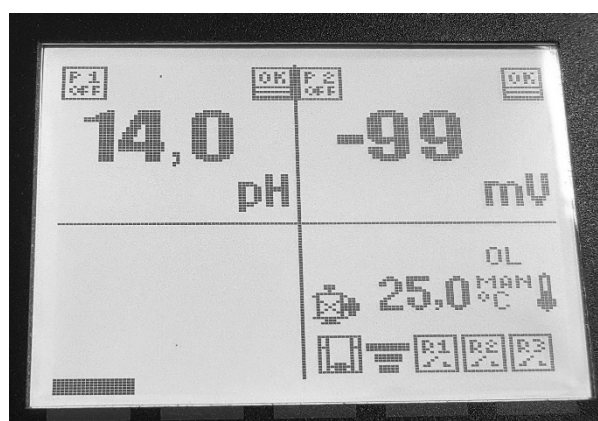
VA DOS BASIC CHLOR (PH / ORP)
