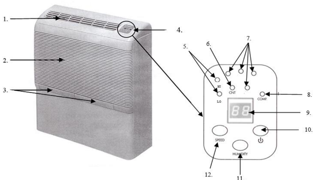
Obrázek č. 1 - popis odvlhčovače a ovládacího panelu
